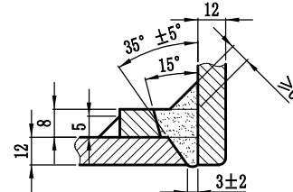
有补强圈接管焊接视图N4
