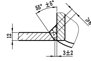
无补强圈接管焊接视图
