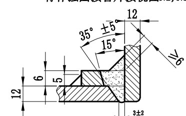
有补强圈接管焊接视图N1, N5
