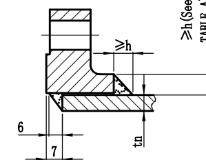
法兰与接管焊接视图
