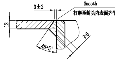
接管N6焊接视图
