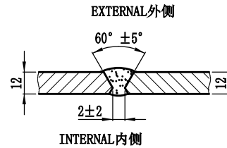
纵环焊缝焊接视图
